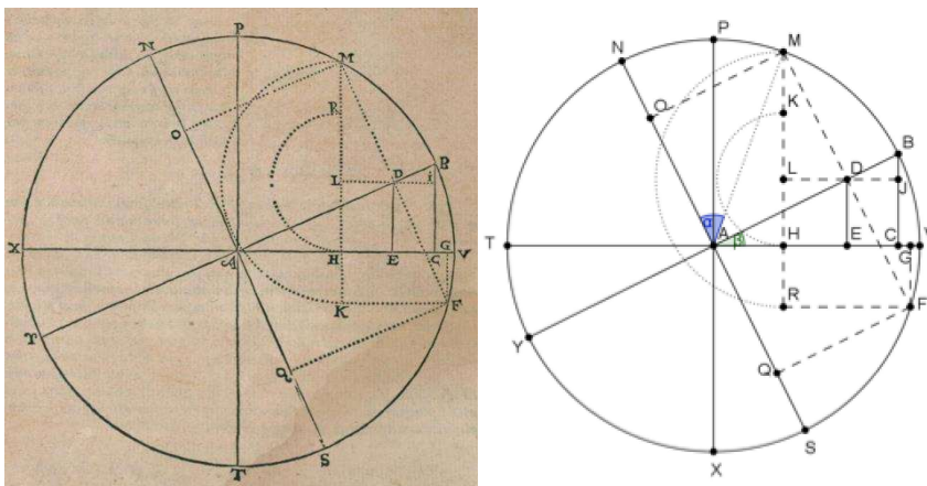
Fig. 1: Prosthaphaeresis-Diagramm aus Nicolaus Reimar Ursus' Fundamentum Astronomicum (Strassburg 1588), p. 16v; und moderne Rekonstruktion mittels Geogebra von M.M.Capalbo, 2017.
