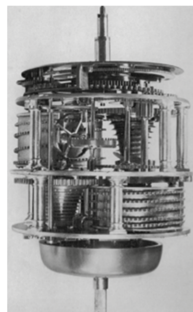
Abbildung 2-5: Uhrwerk des kleinen Himmelsglobus von Jost Bürgi, 1594 (aus [8, S. 45]).
