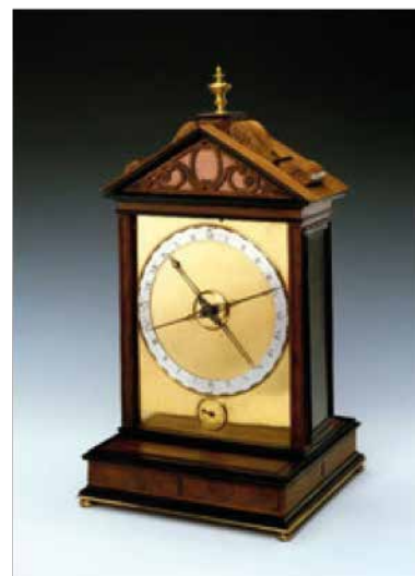
Abbildung 2-4: Sekundenuhr um 1580, wenig Verzierungen, ein Messinstrument.
