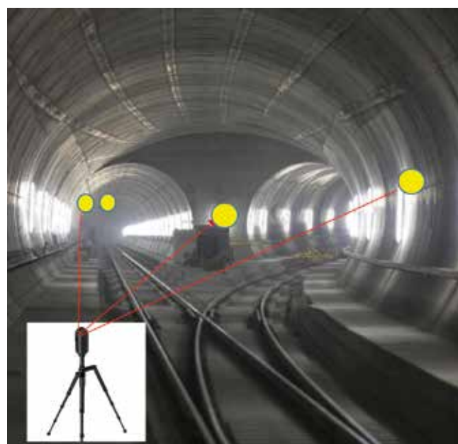
Abbildung 5-11: LOPS Anwendung in Tunneln
