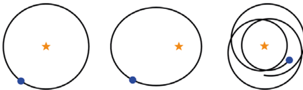
Abbildung 3-1: Beispiele von möglichen Umlaufbahnen eines Planeten um einen Zentralstern: Kreisbahnen (links) oder die aktuelle Ellipsenbahnen der Planeten (Mitte) bilden einfache, geschlossene Kurven. Wenn die Anziehungskraft nur leicht von der Newtonschen Form abweicht (rechts), sind die Kurven nicht mehr geschlossen, und der Planet stürzt irgendwann entweder auf den Stern oder wird ins All geschleudert.
