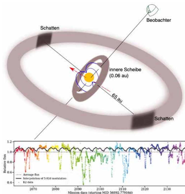
Abbildung 4-3: Oben: Illustration des Systems des jungen Sterns RX-J1604.3-2130A mit Stern, umgebenden Scheiben aus Staub und Gas (nicht massstabsgetreu). Unten: Zeitliche Variation der Lichtintensität des Sterns (Abb. basierend auf Sicilia-Aguilar et al. 2020).
