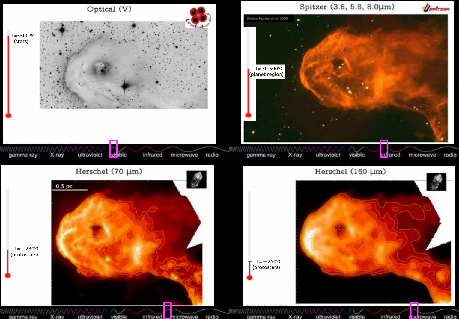
Abbildung 4-2: Der IC1396A sternbildende Nebel gesehen durch verschiedene Teleskope. Verschiedene Wellenlängen geben Überblick über die Regionen des Nebels, oder die Regionen der Sterne und deren protoplanetaren Scheiben, die bestimmte Temperaturen haben. Die Daten wurden als Teil der Forschungsarbeit von A. Sicilia-Aguilar mit dem 3.5 m Calar Alto Teleskop, dem Spitzer Space Telescope und dem Herschel Space Observatory aufgenommen (basierend auf Sicilia-Aguilar et al. 2015).
