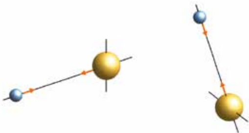
Abbildung 3-4: Illustration der Translations- und Rotationssymmetrie. Ein System von zwei Körpern wird verschoben und gedreht. Die durch die orangenen Pfeile dargestellten Anziehungskräfte zwischen den beiden Körpern hängen nicht von der absoluten Position und Ausrichtung jedes Körpers im Raum ab, sondern nur von deren Abstand voneinander. Die relative Bewegung bleibt unverändert.
