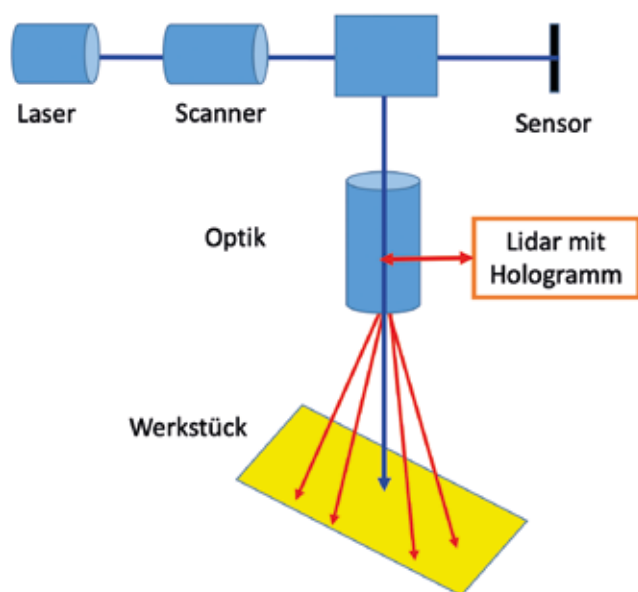
Abbildung 5-13: Das verkippte Werkstück (gelb) soll mit einem Laserstrahl (blau) bearbeitet werden. Das Lidarsystem (rot) erzeugt mit einem Hologramm vier Zielvektoren, aus denen die aktuelle Lage des Werkstücks berechnet werden kann.
