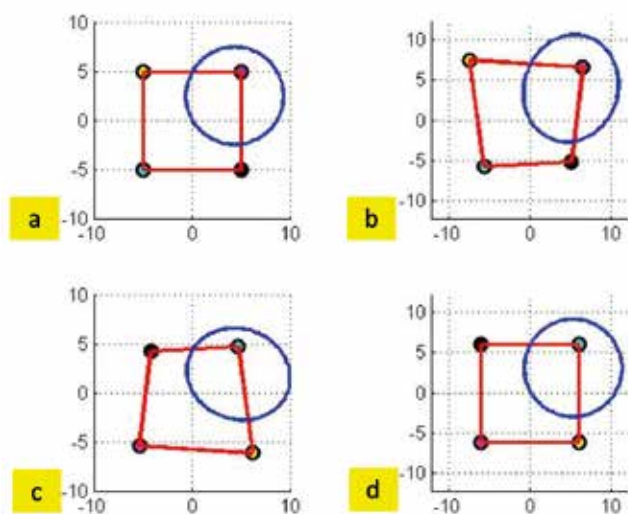
Abbildung 5-14: a) Scannerablenkung, b) Laserfigur auf verkipptem Werkstück, c) korrigierte Scannerablenkung; d) korrigierte Laserfigur auf verkipptem Werkstück
