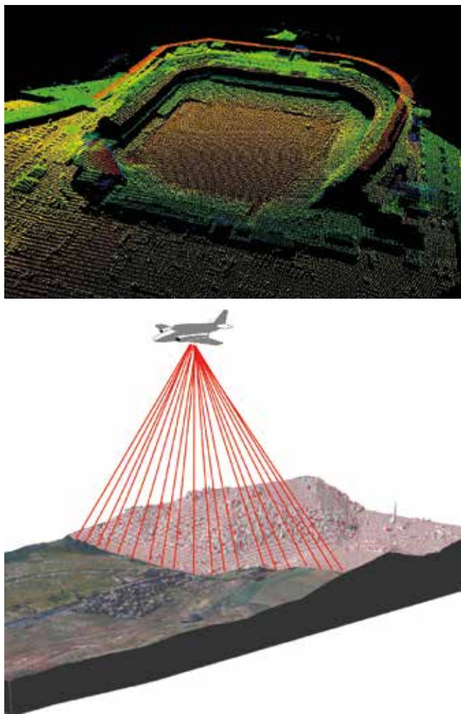
Abbildung 5-12: Scandaten eines überflogenen Sportstadions (oben) und Prinzipweise des Lidarscanners (unten)
