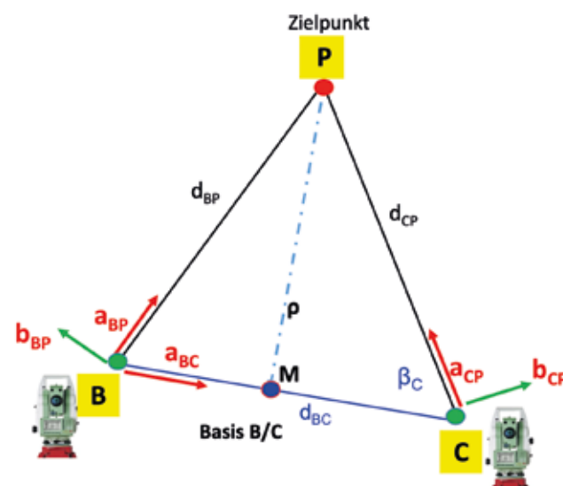
Abbildung 5-15: Triangulationsbasis
